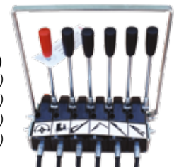
Comando con cavi flessibili (MM.3500) Cable controls (MM.3500) Commandes par cables teleflexibl. (MM.3500) Comandos a distancia teleflexibl. (MM.3500) Flexible Kabelsteuerung (MM.3500)
