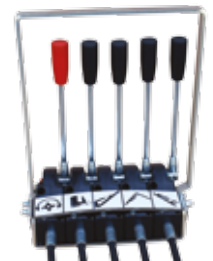
Comando con cavi flessibili (MM.3000) Cable controls (MM.3000) Commandes par cables teleflexibl. (MM.3000) Comandos a distancia teleflexibl. (MM.3000) Flexible Kabelsteuerung (MM.3000)
